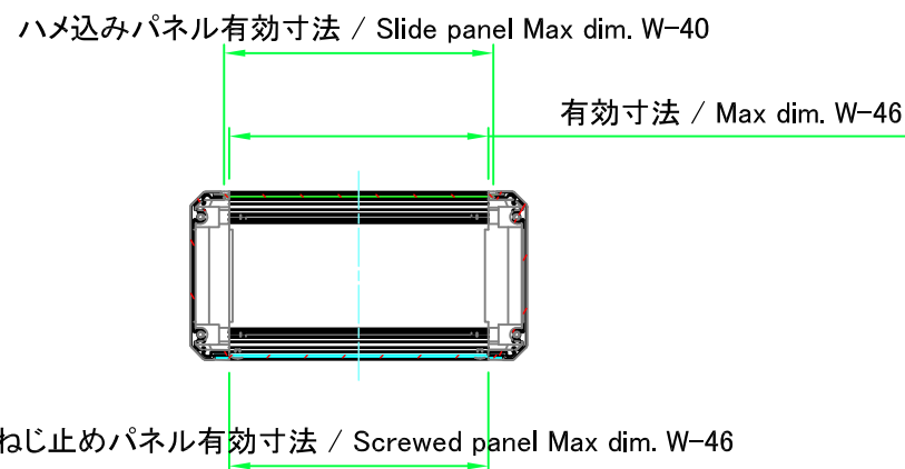
A-A ( 1 : 5 )
